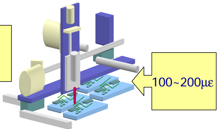
切割 Routing
